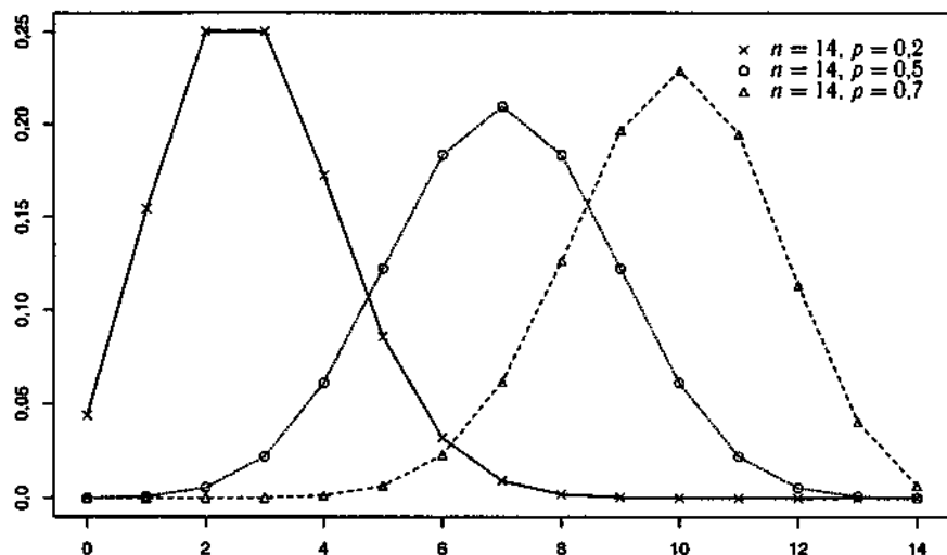
Рис. 1.3. Биномиальное распределение
