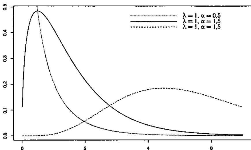
Рис. 2.7. Плотности гамма-распределения
